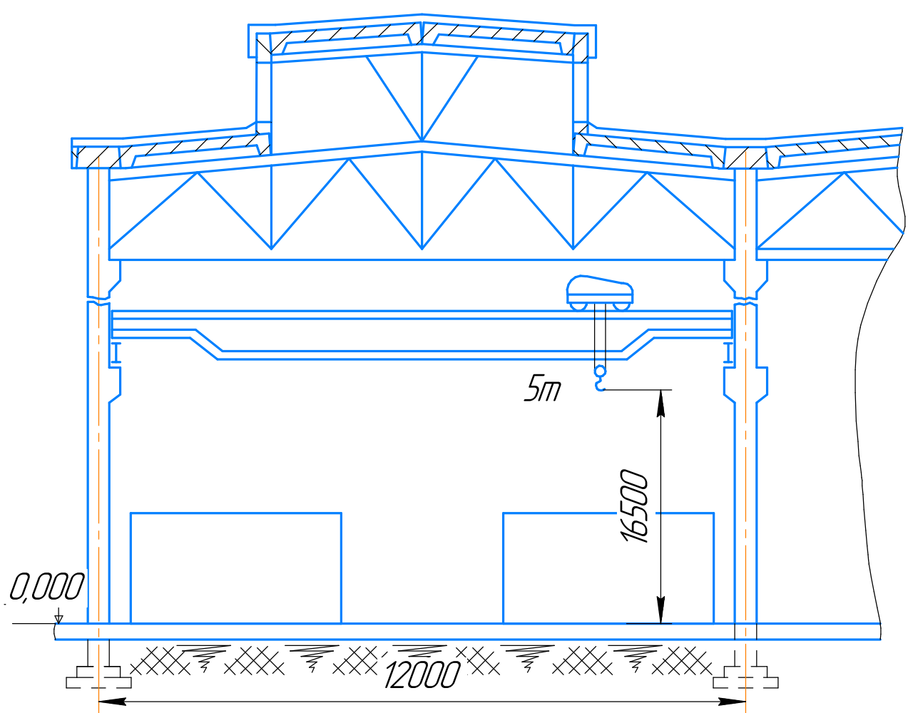
А-А (1:100)
